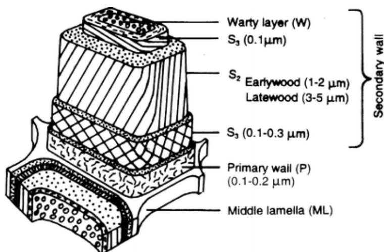
Abbildung 15: Schematische Darstellung einer Holzzeile
