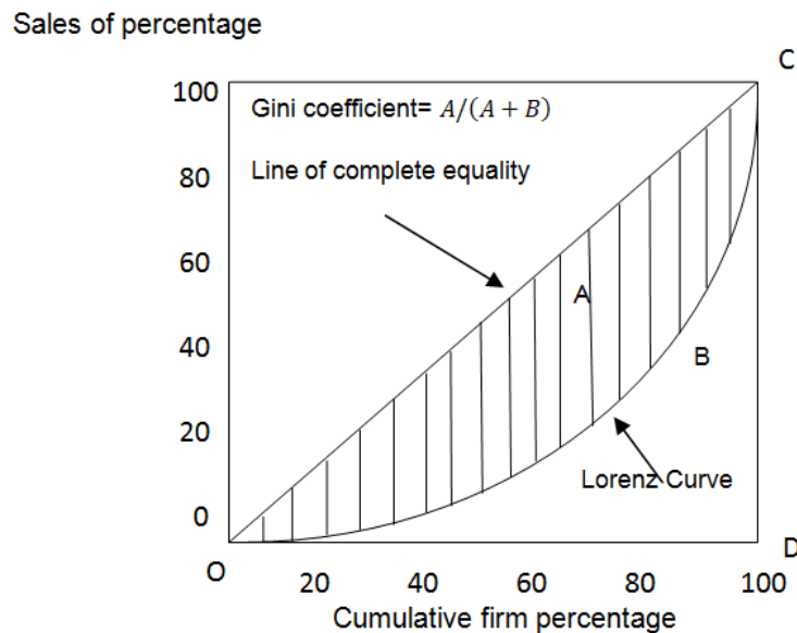
Fig. 2. Lorenz Curve
