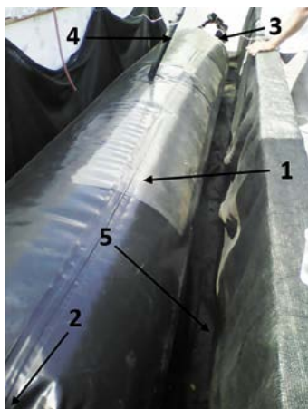
Figura 1. Aspecto general del biodigestor tubular de geomembrana: 1: Cuerpo del biodigestor, 2: Alimentación del afluente, 3: Salida del efluente, 4: Salida del biogás al reservorio, 5: Pileta con cubierta.
