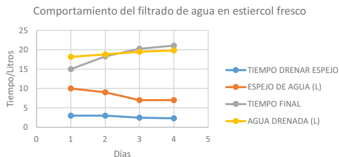
Figura 10. Comportamiento del filtrado de agua en estiércol fresco.
