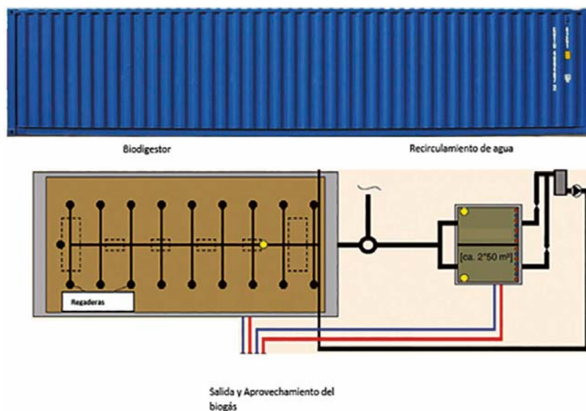
Figura 12. Diagrama del diseño conceptual del biodigestor. Vista de arriba interna y lateral externa.
