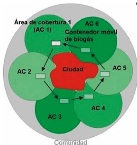
Figura 6. Diagrama de optimización de almacén y transporte para el primer esquema de recolección de residuos orgánicos de manera descentralizada.
