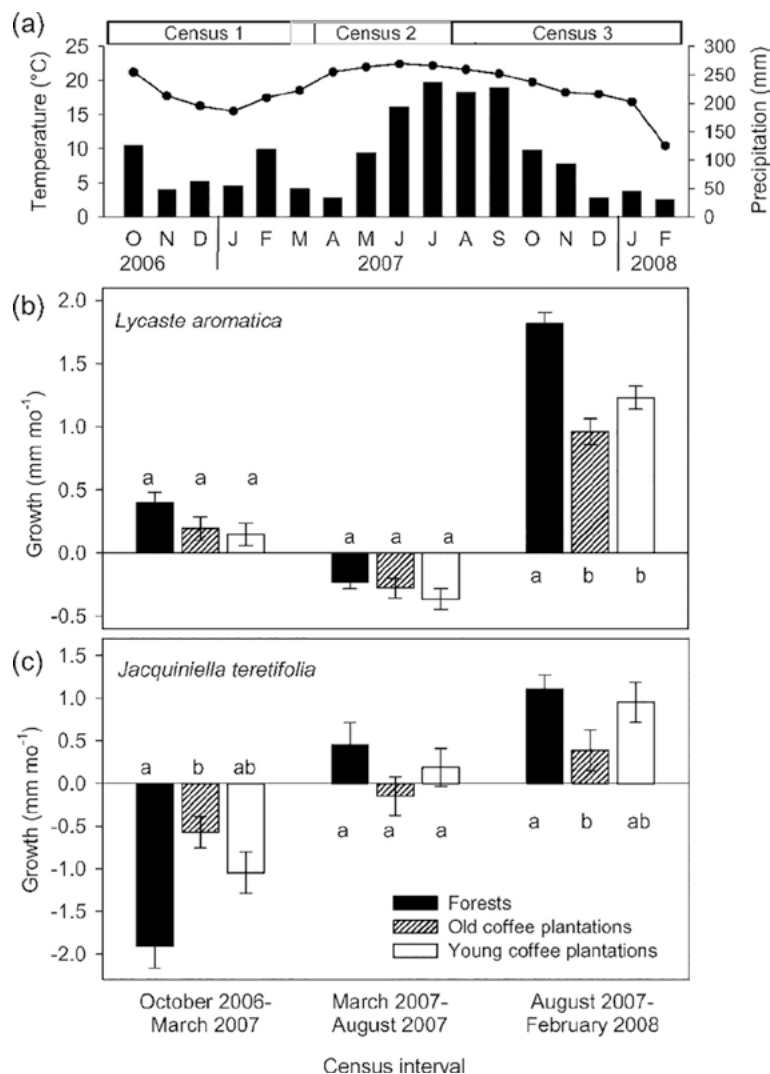
Figura 1. Datos climáticos mensuales (a) y crecimiento semestral de Lycaste aromatica (b) y Jaquiniella teretifolia (c) en un bosque y dos cafetales en el centro de Veracruz (tomado de Scheffknecht et al. 2010).
