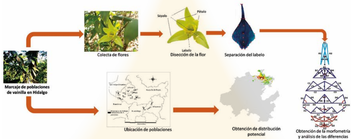
Figura 1. Metodología para la determinación de la distribución potencial e identificación del germoplasma de Vanilla planifolia Jacks. ex Andrews en Hidalgo, México.
