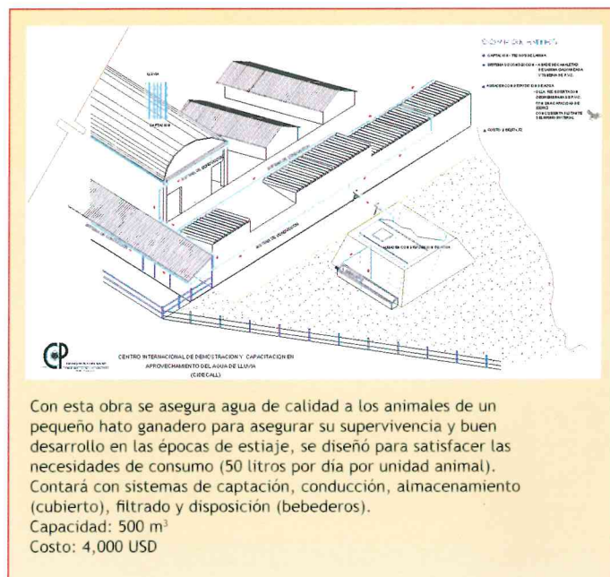
Figura 4. COLPOS 4. Abrevadero para pequeñas explotaciones ganaderas.
