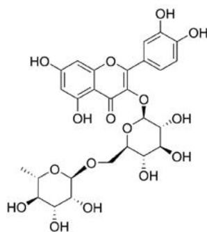
Rutin
