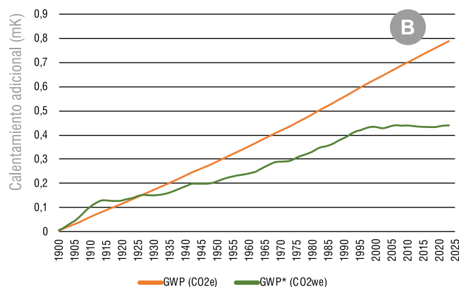
Figura 2 - Dinámica de emisiones anuales como CO 2 e (GWP) y CO 2 we (GWP*) (izquierda) y contribución acumulada al calentamiento (mK) (B), 1900-2023.
