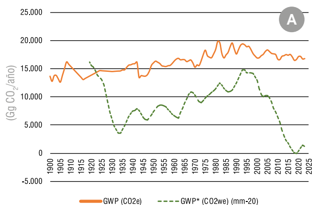
Figura 2 - Dinámica de emisiones anuales como CO 2 e (GWP) y CO 2 we (GWP*) (izquierda) y contribución acumulada al calentamiento (mK) (B), 1900-2023.
