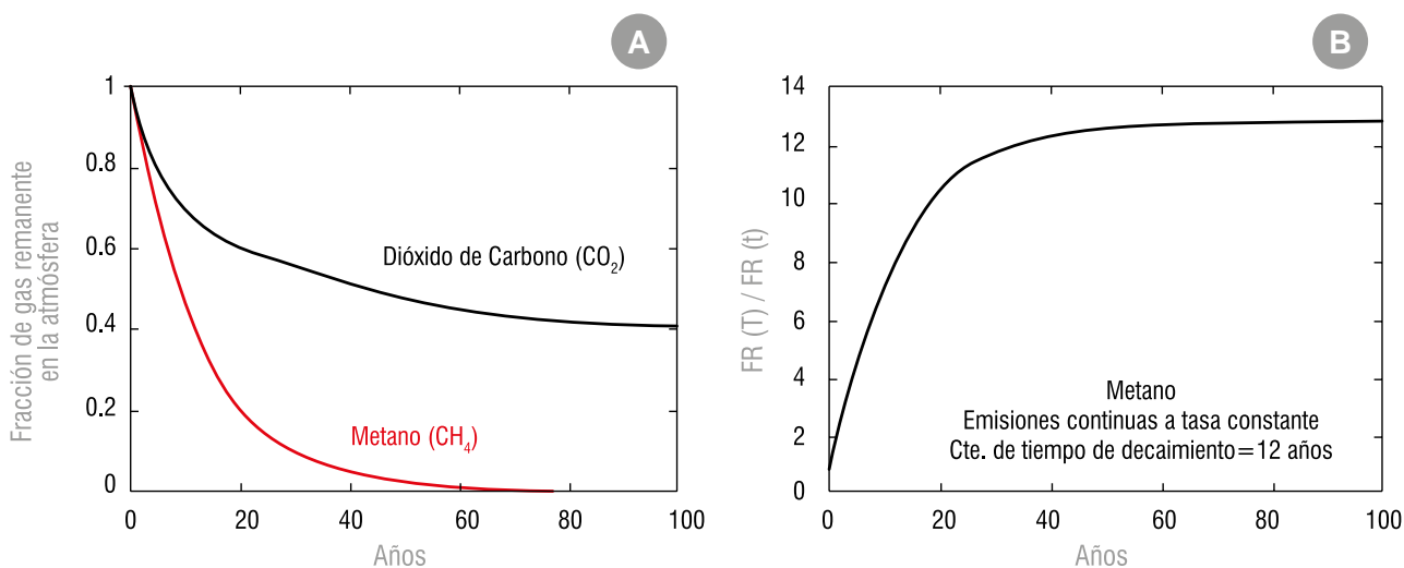
Figura 1 - Decaimiento atmosférico de \text{CH}_4 y \text{CO}_2 luego de un pulso de emisión en el año cero (A) y saturación del FR de \text{CH}_4 como resultado de emisiones continuas a tasa constante (B). Fuente: Kleinberg, 2020
