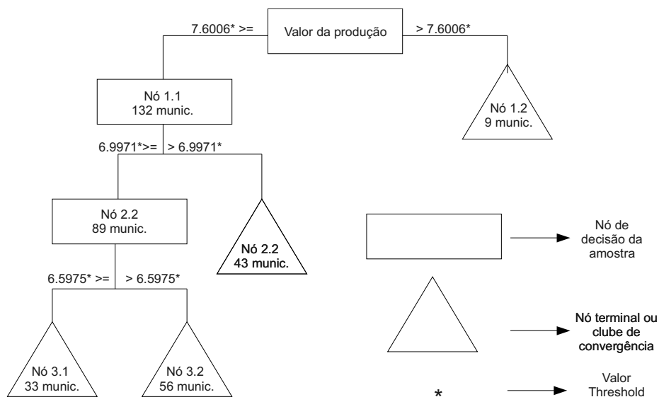
Figura 8. Diagrama de decisão do efeito threshold
