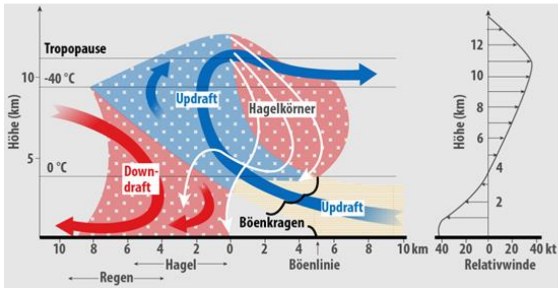
Abbildung 5-3: Schema einer Gewitterwolke (Quelle: DWD).
