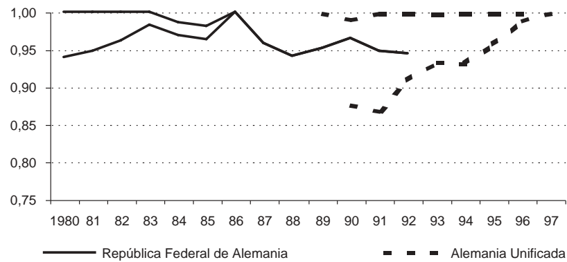
Figura 3. Límites de eficiencia radial. Alemania.
