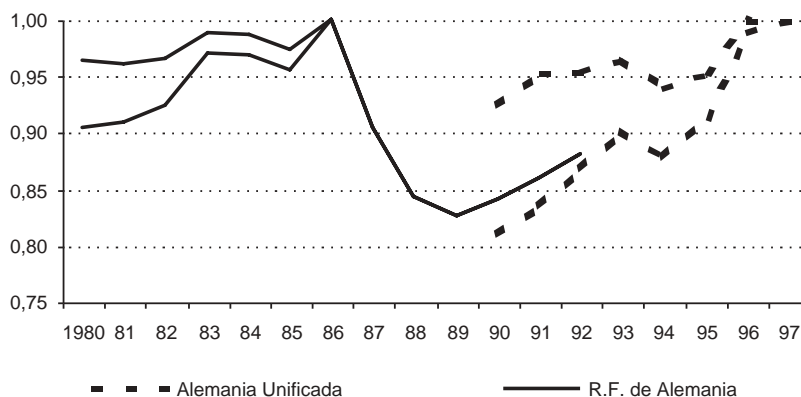
Figura 4. Límites de eficiencia de Otros Consumos Intermedios. Alemania.
