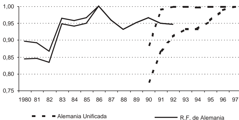
Figura 5. Límites de eficiencia de Trabajo. Alemania.
