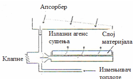
Слика.6. Соларна сушара са допунским извором енергије и сушењем материјала у слоју
