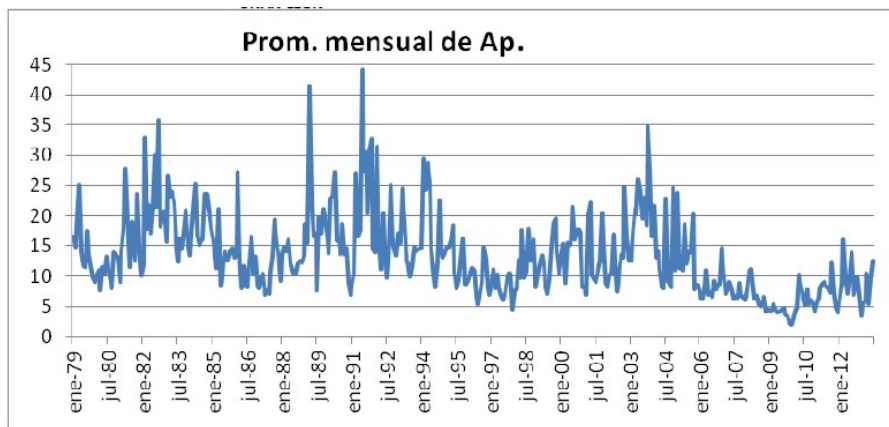
FIGURA 2A Series de tiempo índice geomagnético Ap (a), de la producción de miel (Tm) (b),cera (Kg)(c), rendimiento por colmena (Kg/colmena)(d) . En todos los casos son promedios mensuales. La serie comienza en enero de 1979 y concluye en marzo del 2013. Promedio mensual de Ap (a)
