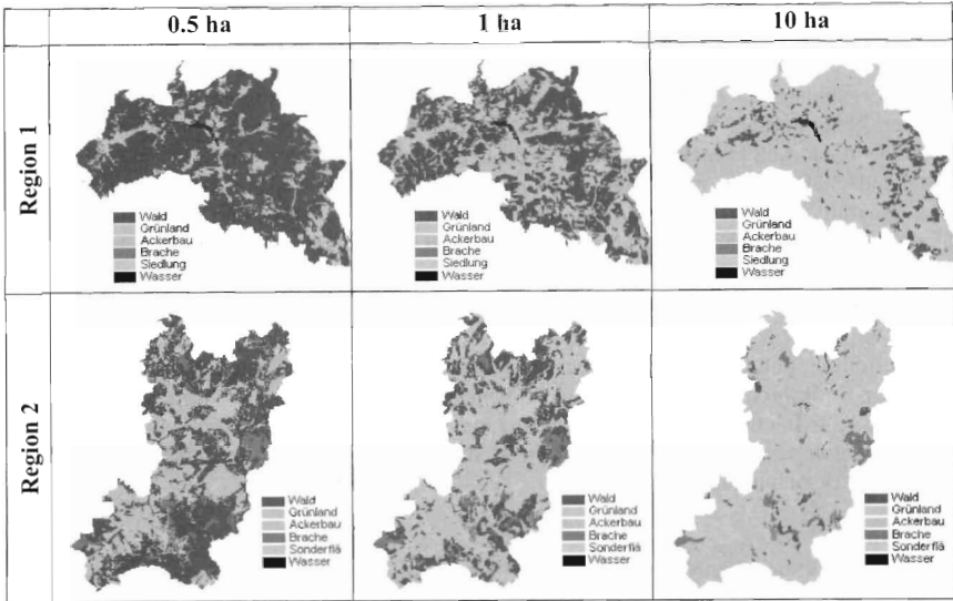
Abbildung 1: Räumliche Auswirkungen zunehmender durchschnittlicher Schlaggrößen
