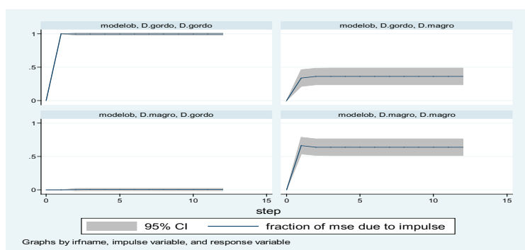
Figura 1 – Decomposição da variância
