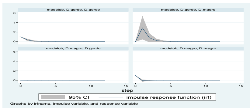
Figura 2 – Função impulso resposta das séries temporais analisadas FONTE: Dados baseados na Seab e IEA (2012)
