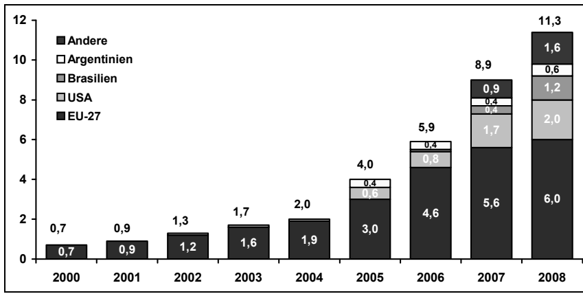
Abbildung 13. Globale Biodieselpromotion in Mio. Tonnen
