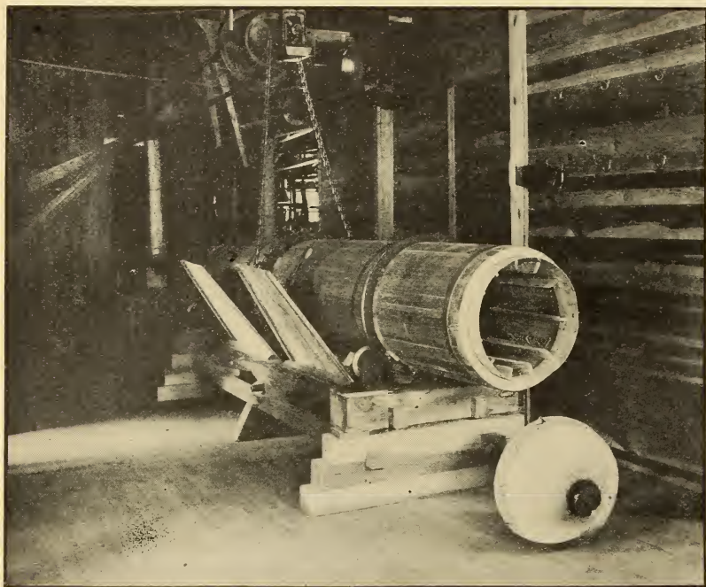
FIG. 9.—Attritionizer.
