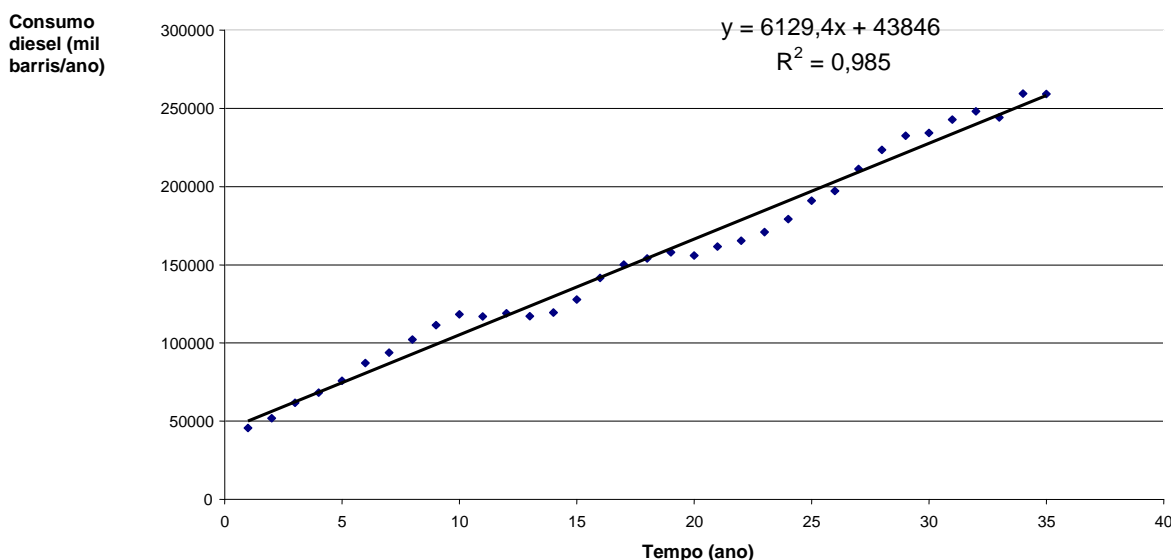
Gráfico 1 – Regressão do consumo de diesel em função do tempo
