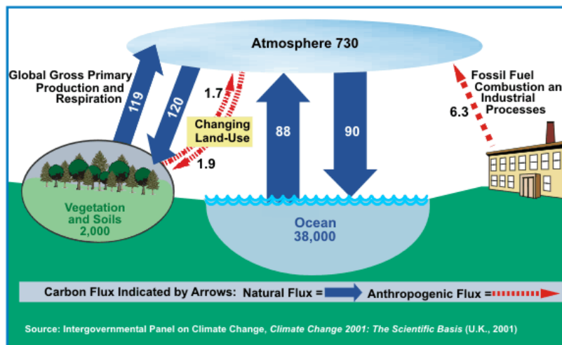
Figura 1 – Ciclo global do Carbono
