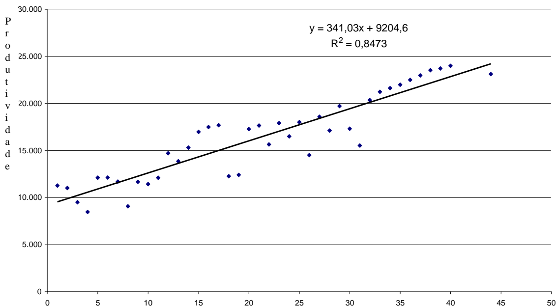
Gráfico 2 – Regressão da produtividade da soja em função do tempo
