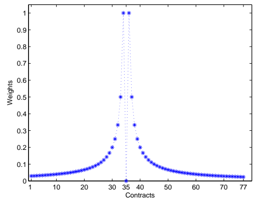
(d) w_{35}
