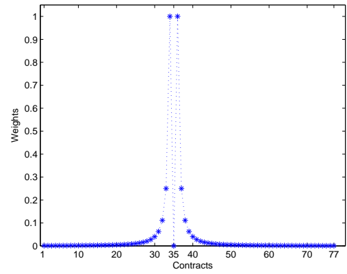
(b) w^1
