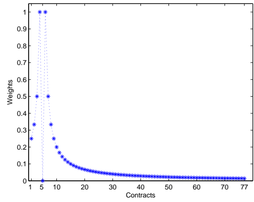
(b) w_5
