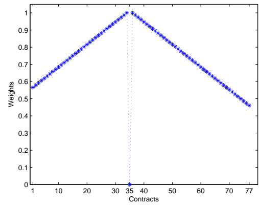
(d) w^3
